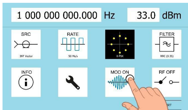
Рис. 25. Включение/выключение модуляции
